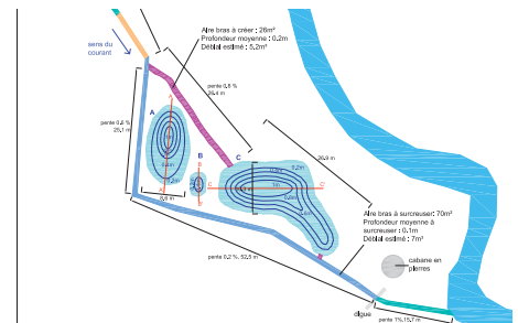
Plan de l'aménagement des étangs.
